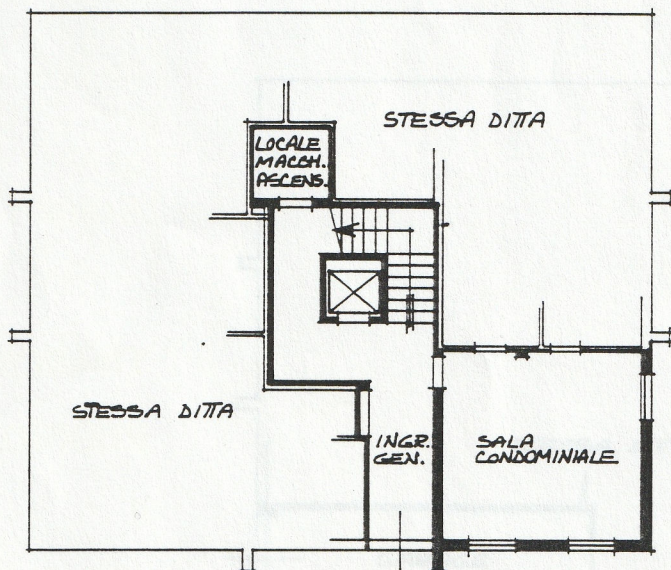
PIANO TERRA H = 2.50 m.
