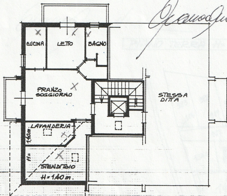
PIANO TERZO H = 2.70 m.
